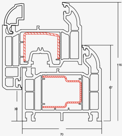
O70 OVOLO PROFILE
